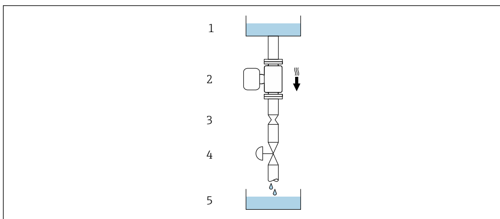
18 Монтаж в трубе с нисходящим потоком (например, для дозирования)
