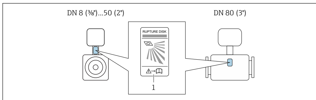
20 Этикетка разрывного диска
