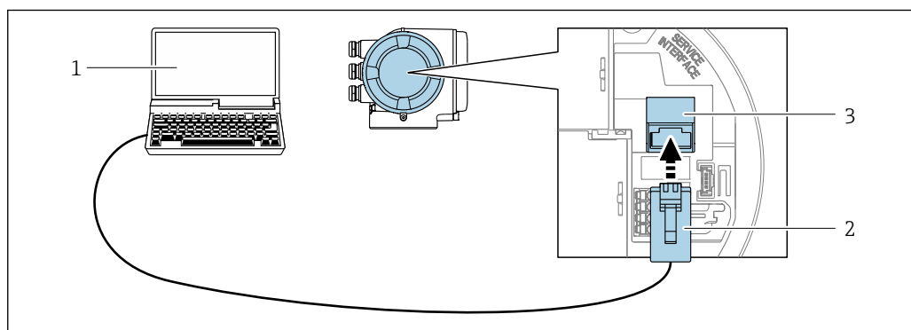
44 Подключение через служебный интерфейс (CDI-RJ45)
