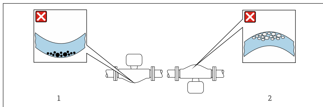
☒ 19 Ориентация сенсора с изогнутой измерительной трубой
