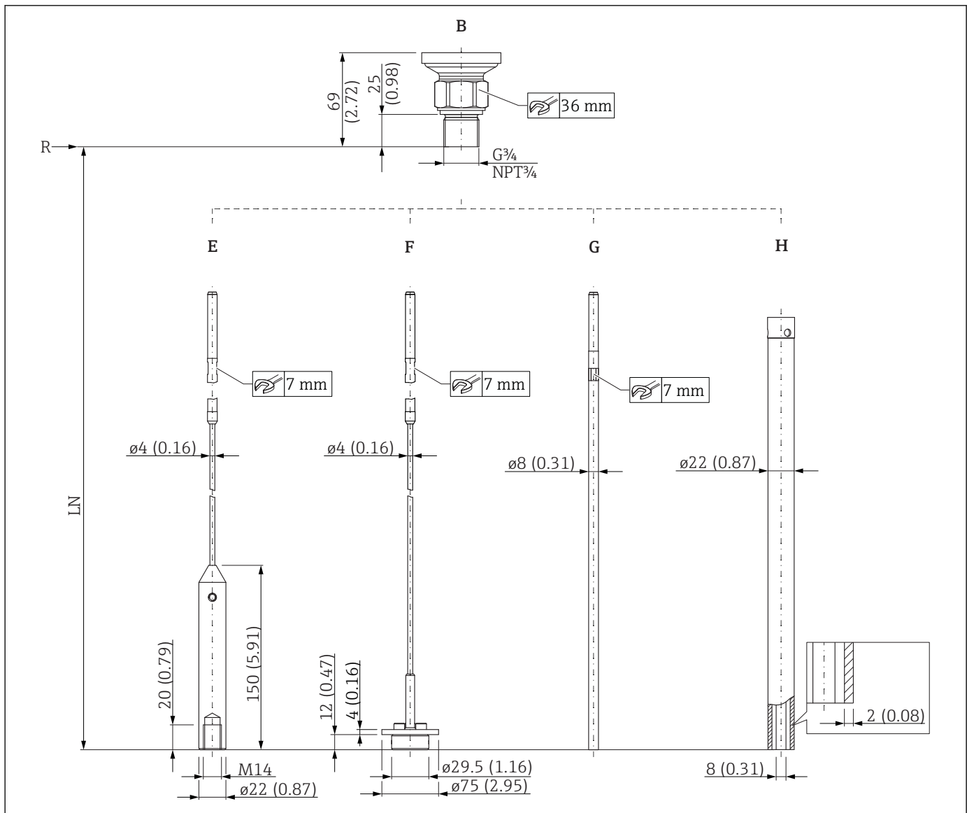
36 FMP51: присоединение к процессу/зонд. Единица измерения мм (дюйм)
