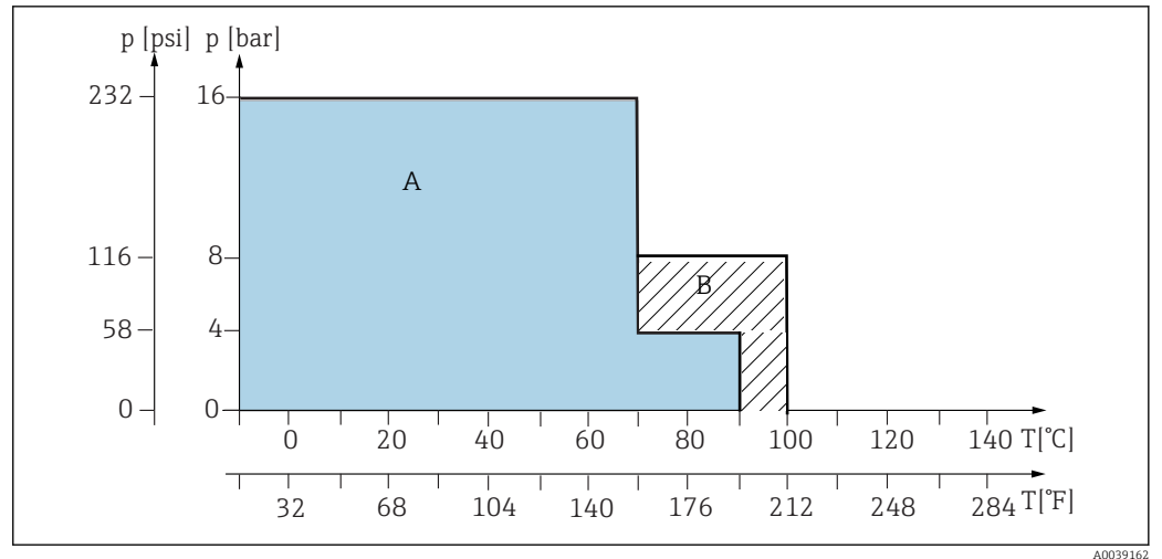
11 Кривые зависимости температура/давление для базового исполнения для материалов PVDF и электропроводящего PVDF
