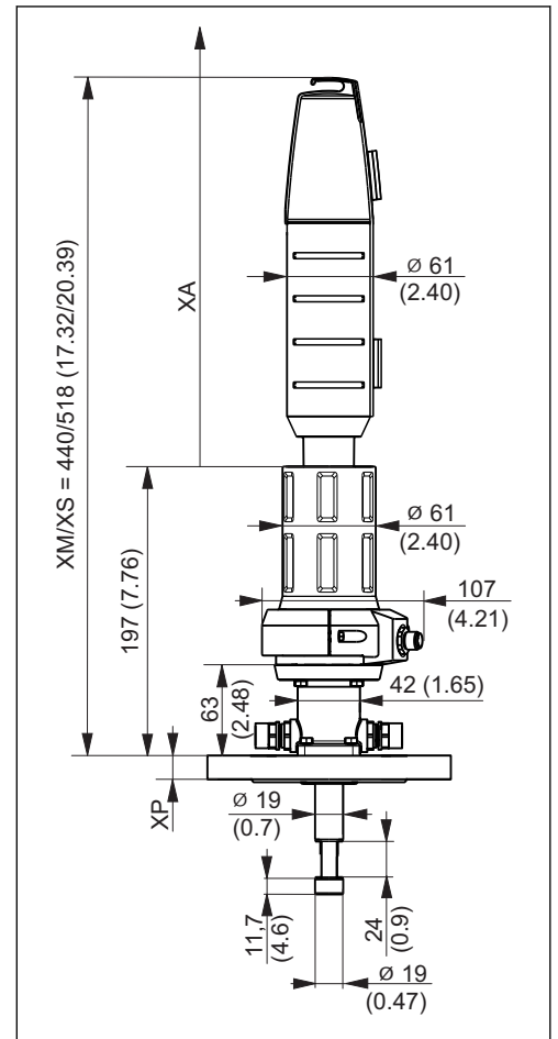
15 Ручной привод, удлиненное исполнение, размеры в мм (дюймах)
