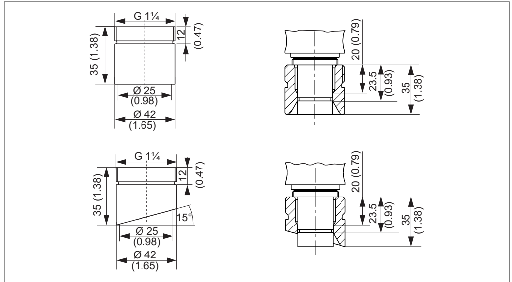
■ 23 Приварной адаптер (предохранительный патрубок), размеры в мм (дюймах)
