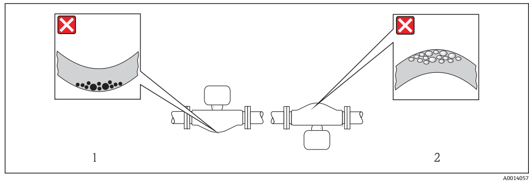
☑ 9 带弯测量管的传感器安装方向示意图
