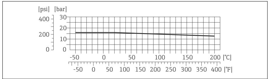
23 连接部件材料: 1.4404 (316/316L)
