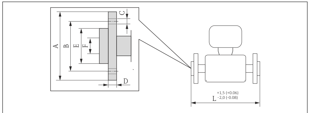
25 单位: mm (in)
