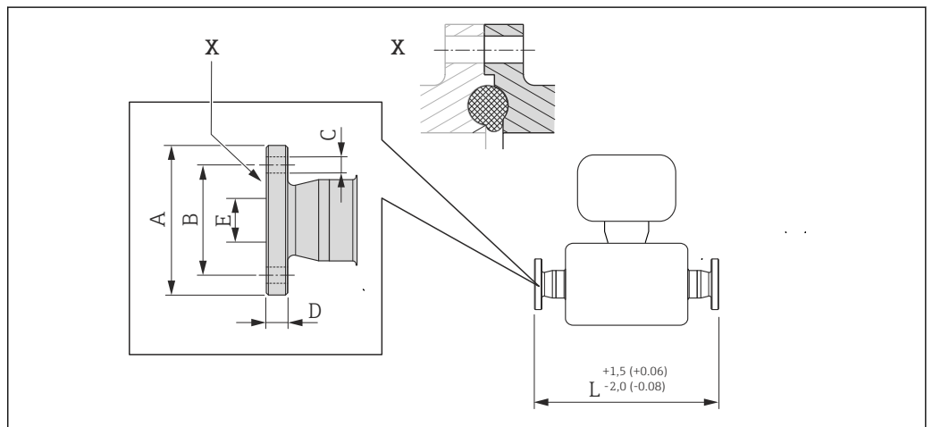
图 34 视图 X: 非对称过程连接; 灰色阴影部分由用户自备。单位: mm (in)
