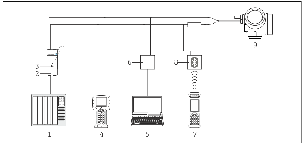
图 44 通过 HART 通信进行远程操作
