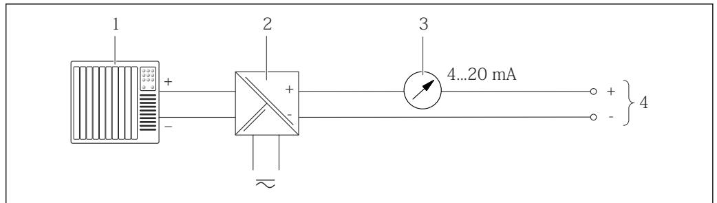
图 2 4...20 mA 无源电流输出的连接示例
