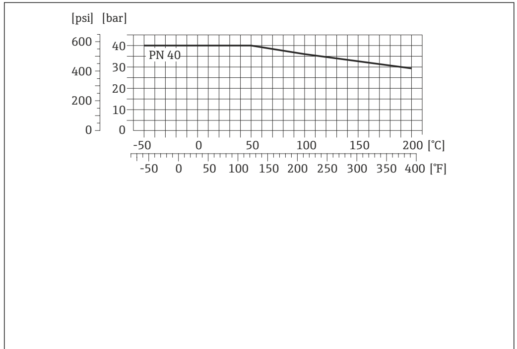
15 法兰材料: 1.4301 (F304); 接液部件材料: Alloy C22 合金
