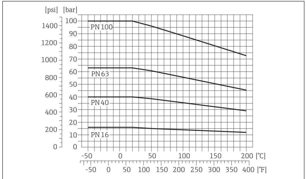
图 11 法兰材料: 1.4404 (F316/F316L)、Alloy C22 合金
