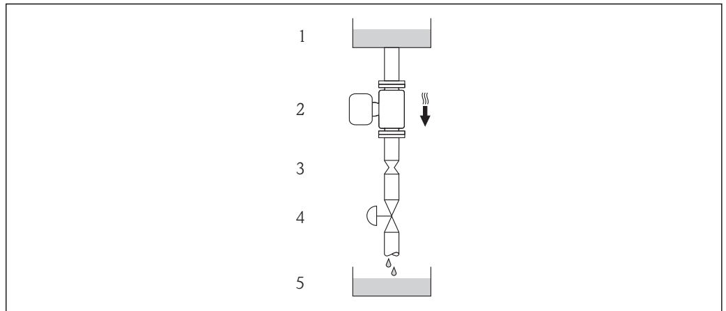
图 8 在向下排空管道中安装(例如: 批量应用场合)
