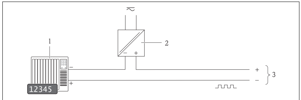
图 3 脉冲/频率输出(无源信号)的连接示例
