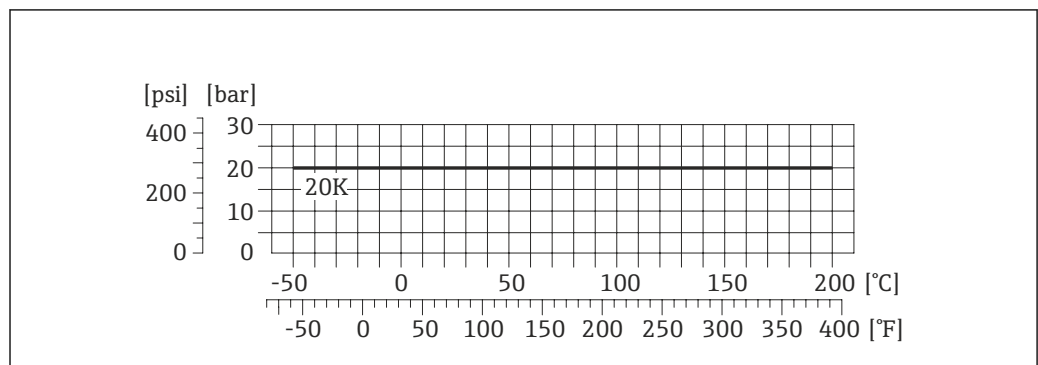
图 17 法兰材料: 1.4301 (F304); 接液部件材料: Alloy C22 合金
