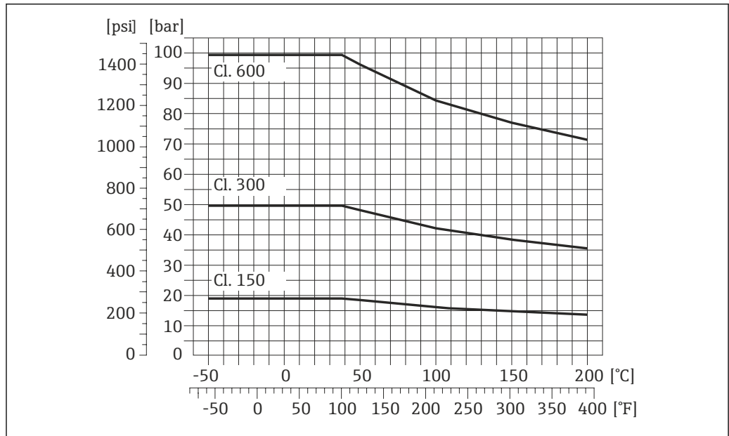
图 13 法兰材料: 1.4404 (F316/F316L)
