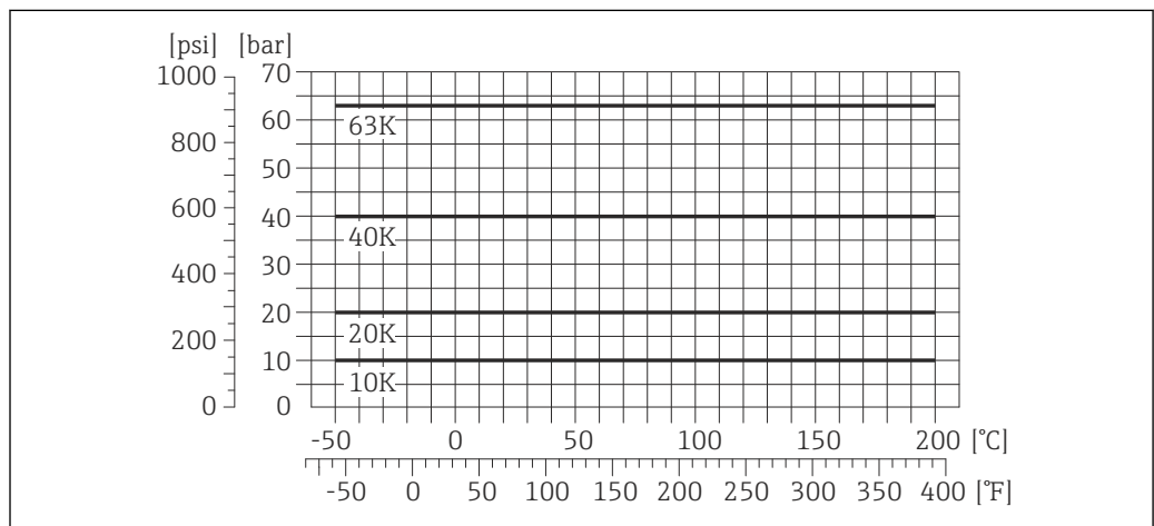
图 14 法兰材料: 1.4404 (F316/F316L)、Alloy C22 合金
