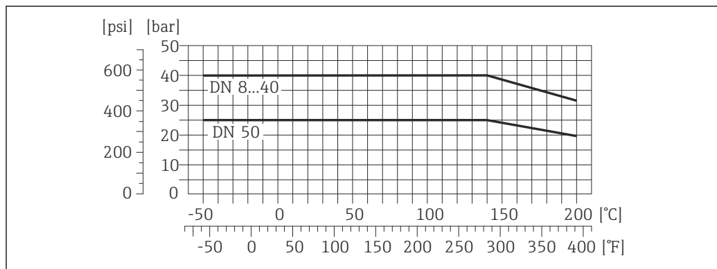
图 21 连接部件材料: 1.4404 (316/316L)
