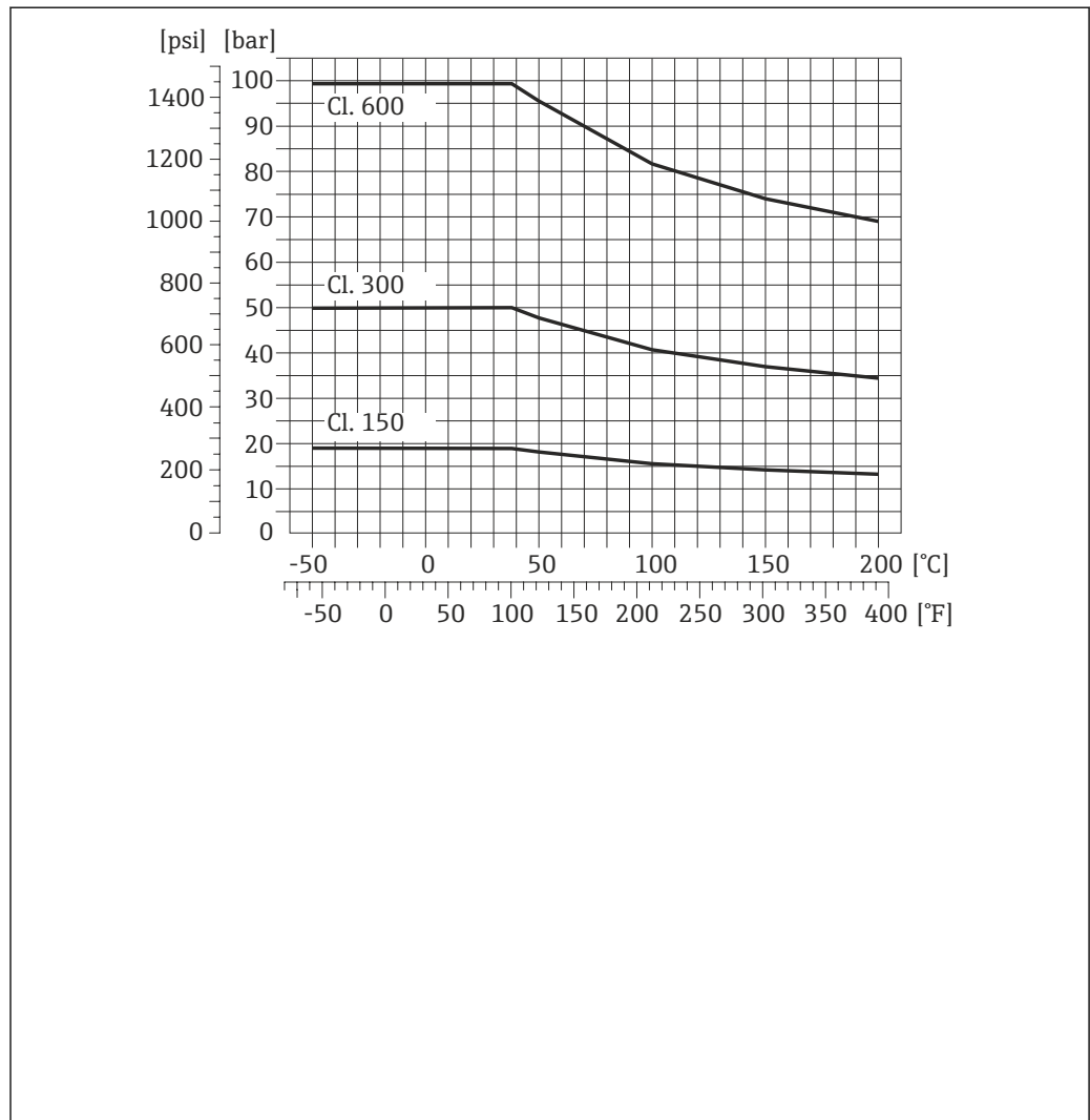
图 16 法兰材料: 1.4301 (F304); 接液部件材料: Alloy C22 合金
