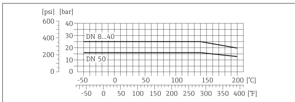
图 22 连接部件材料: 1.4404 (316/316L)
