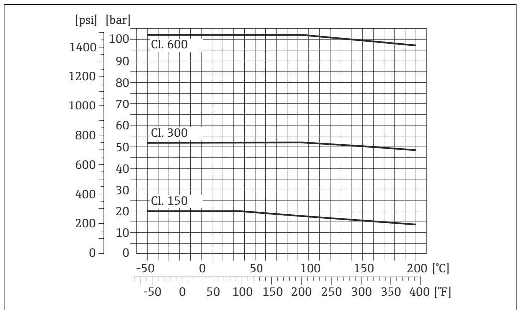
图 12 法兰材料: Alloy C22 合金
