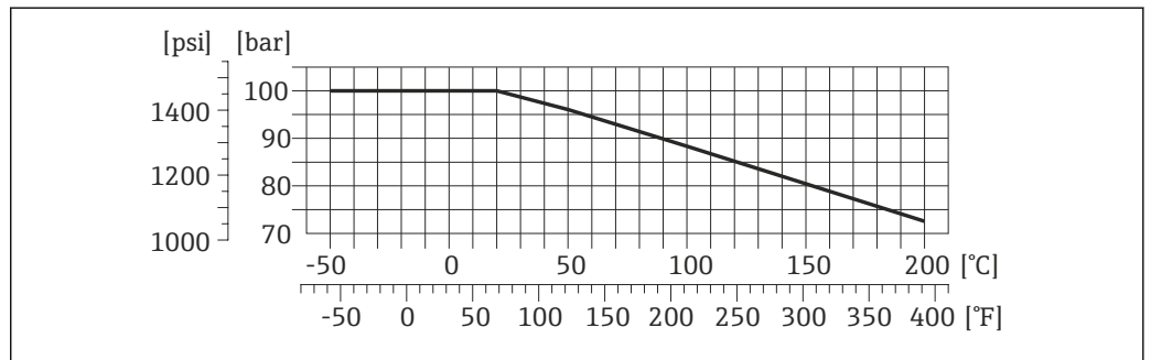
☑ 18 连接部件材料: 1.4404 (316/316L)
