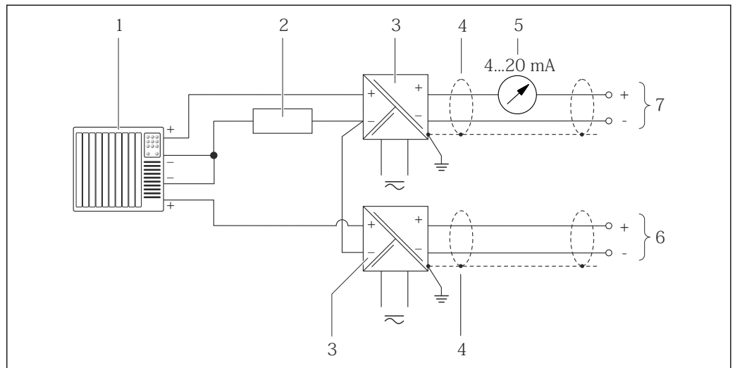
图 7 带公共负端的 HART 输入的连接示例
