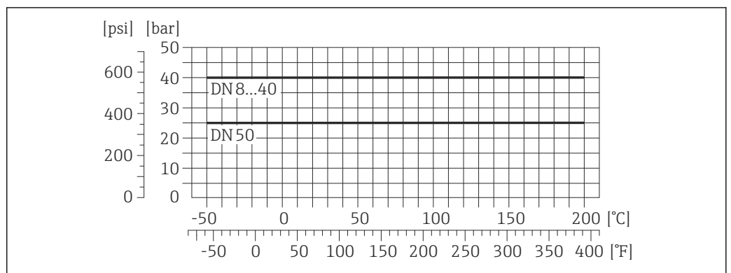
☑ 19 连接部件材料: 1.4404 (316/316L)
