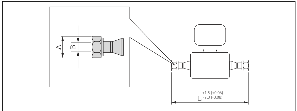
30 单位: mm (in)
