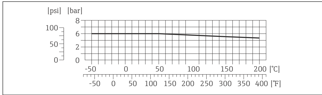
图 20 连接部件材料: 1.4404 (316/316L)
