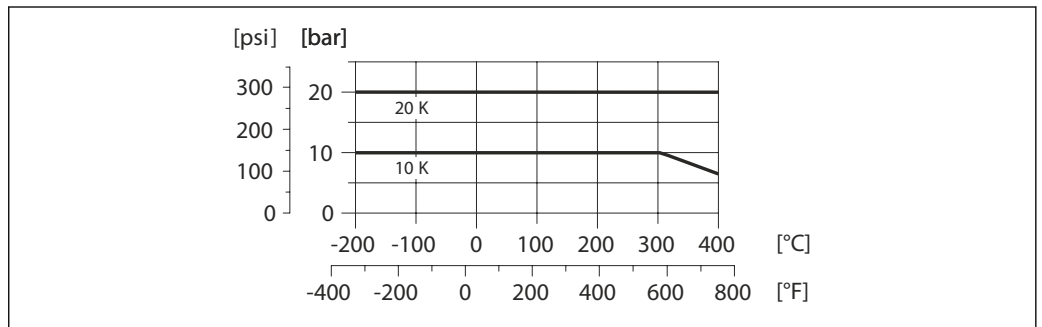
图 19 过程连接材料: 不锈钢, 铸钢, 多项认证, 1.4408 (CF3M)
