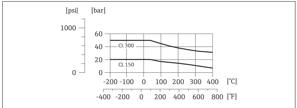
图 18 过程连接材料: 不锈钢, 铸钢, 多项认证, 1.4408 (CF3M)
