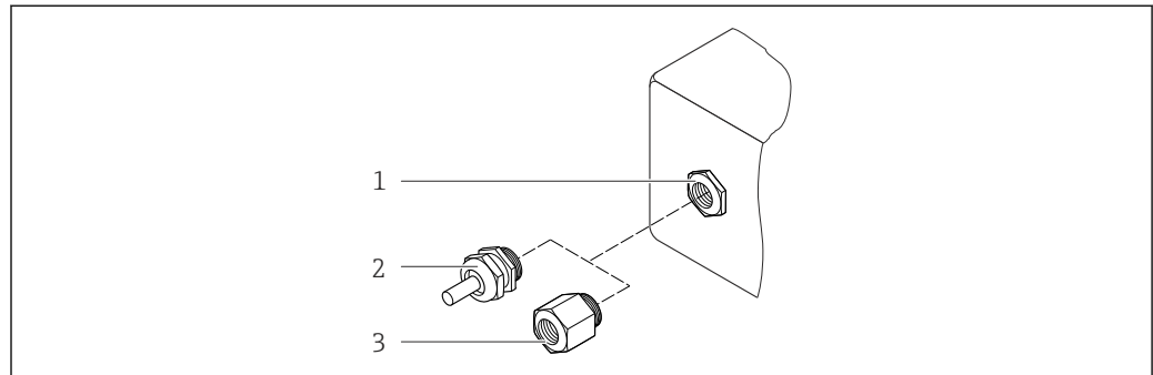
图 22 可能的电缆入口/缆塞
