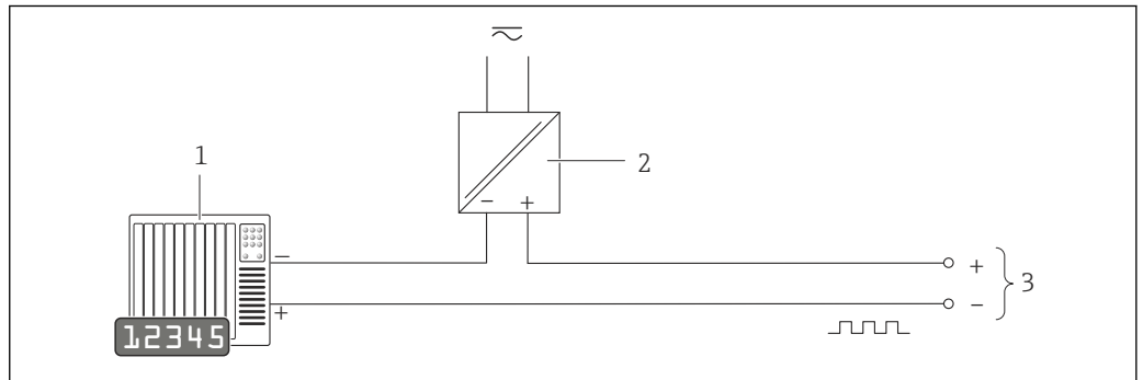
图 6 脉冲/频率输出(无源信号)的连接示例
