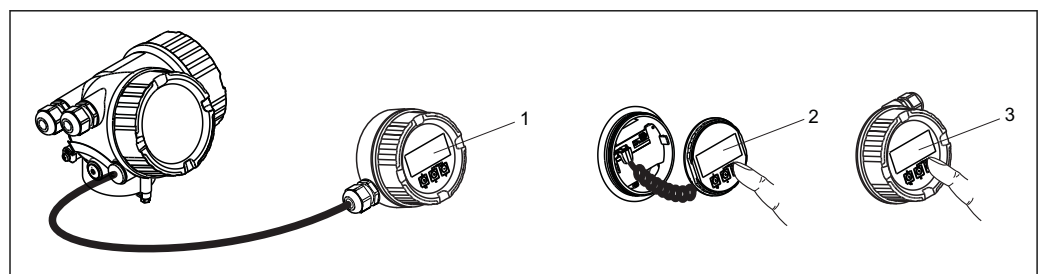
图 23 通过 FHX50 操作的操作选项
