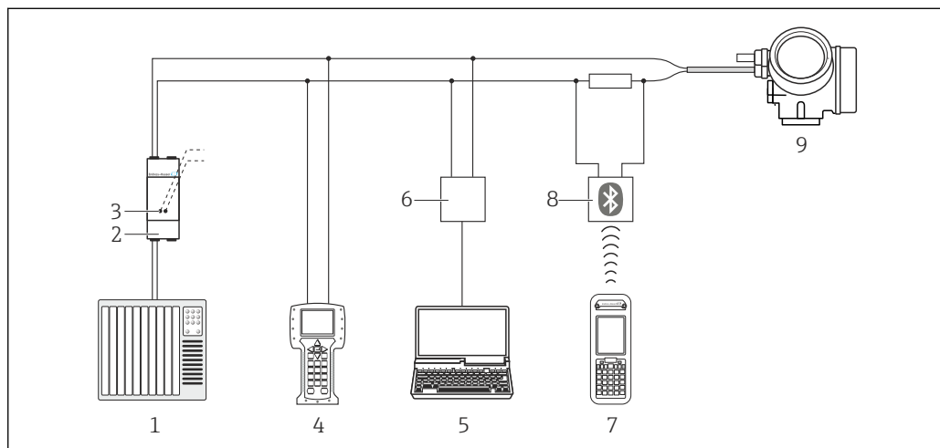
图 24 通过 HART 通信进行远程操作
