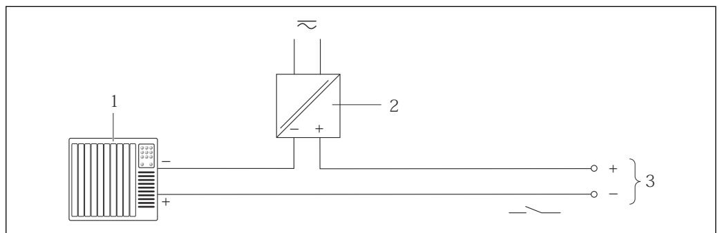
图 7 开关量输出(无源信号)的连接示例
