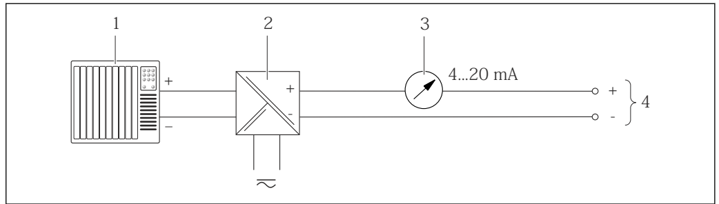
图 5 4...20 mA 无源电流输出的连接示例
