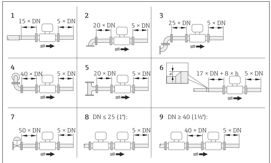
图 12 不同节流装置的最小前/后直管道长度示意图
