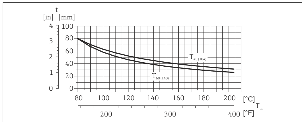
图 29 推荐保温层厚度，取决于介质温度和环境温度
