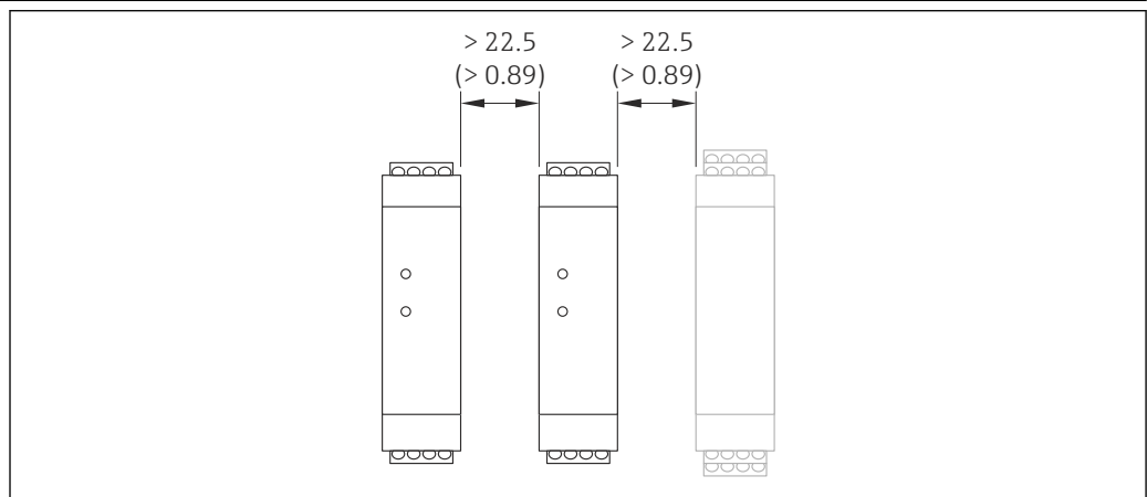
19 Promass100 安全栅或其他模块间的最小安装距离。单位：mm (in)
