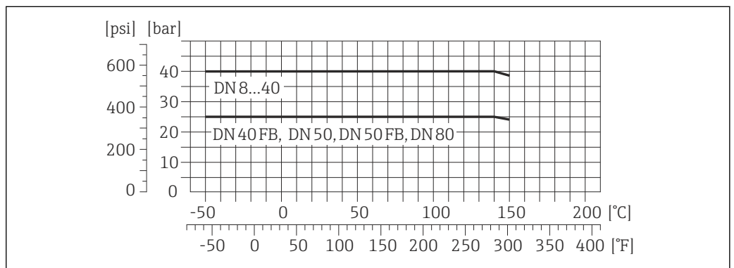
图 25 连接部件材料: 钛
