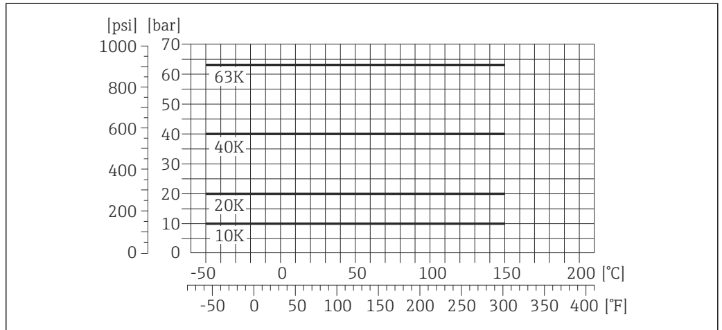
图 23 法兰材料: 1.4301 (304); 接液部件材料: 钛
