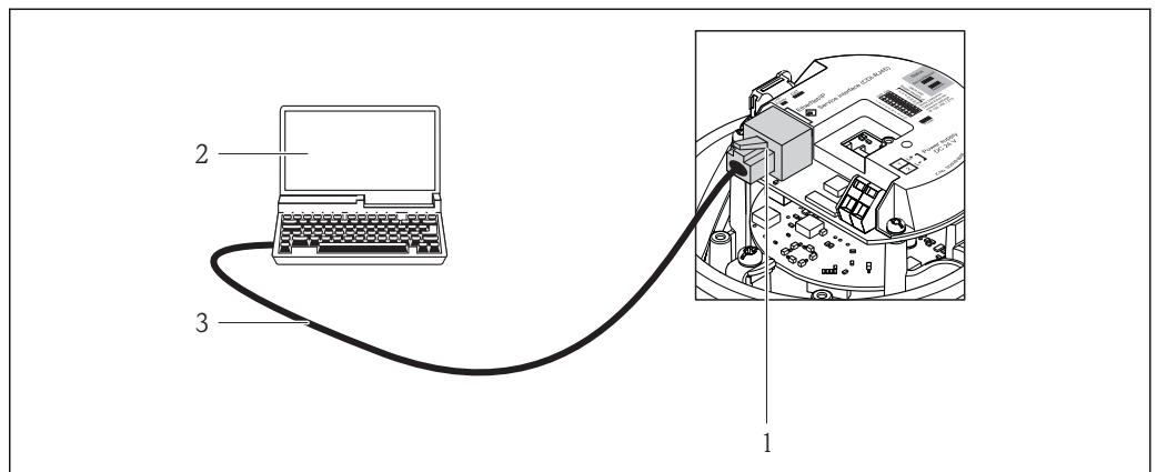
☑ 48 订购选项“输出”，选型代号 N: 工业以太网(EtherNet/IP)
