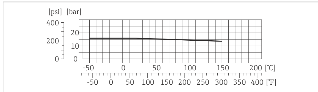
图 27 连接部件材料: 钛
