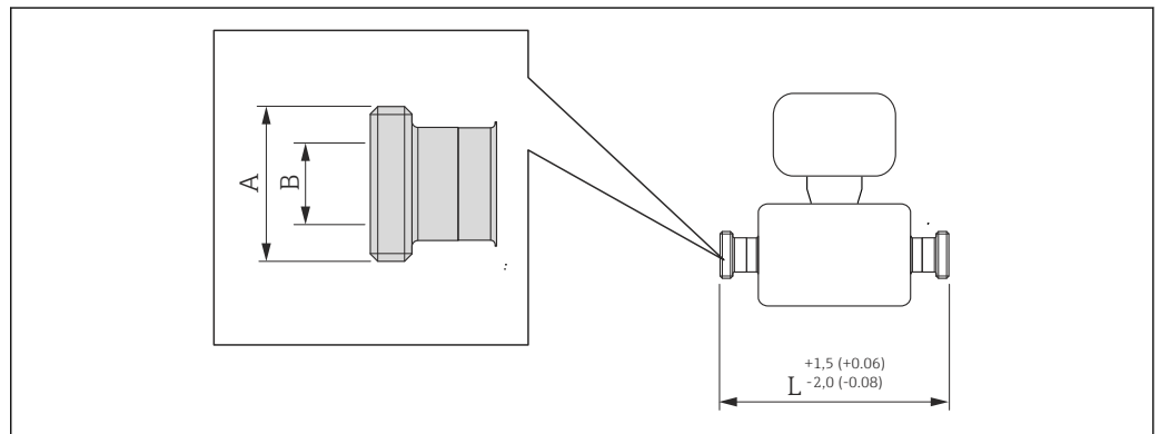
39 单位: mm (in)
