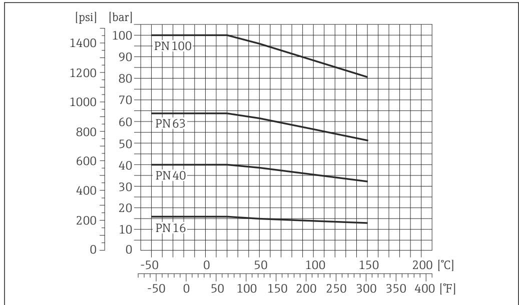
图 21 法兰材料: 1.4301 (304); 接液部件材料: 钛
