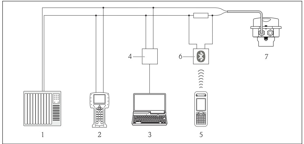
图 45 通过 HART 通信进行远程操作
