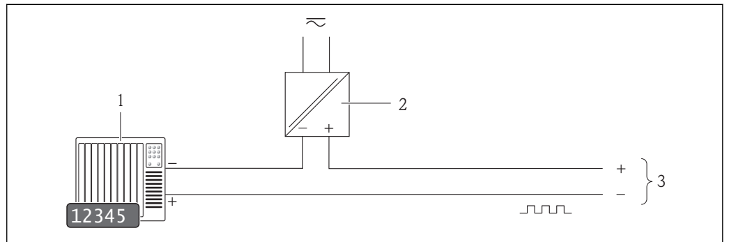
图 9 脉冲/频率输出的连接示例(无源信号)
