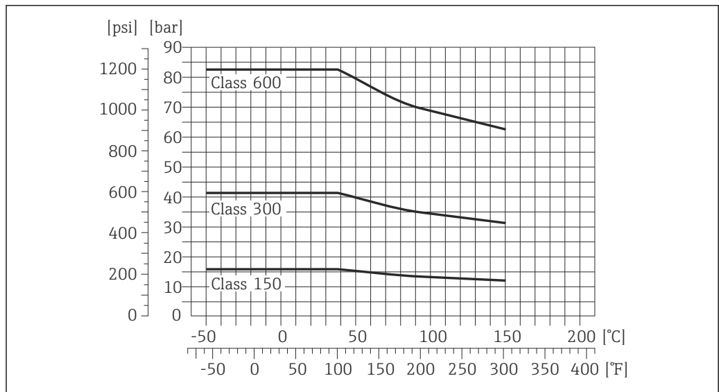
图 22 法兰材料: 1.4301 (304); 接液部件材料: 钛
