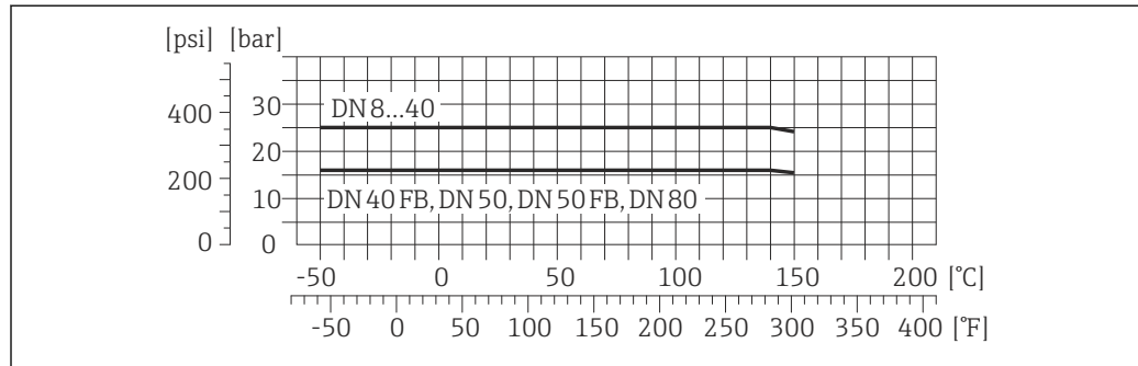
图 26 法兰材料: 钛
