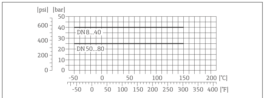
图 24 连接部件材料: 钛
