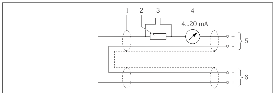
图 15 HART 输入(burst 模式)的连接示例, 通过电流输出(有源信号)
