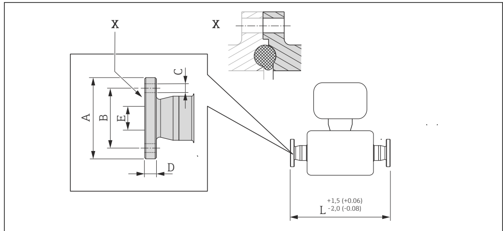
图 37 视图 X: 非对称过程连接; 灰色阴影部分由用户自备。单位: mm (in)
