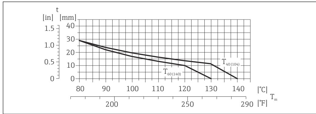
图 28 推荐保温层厚度，取决于介质温度和环境温度
