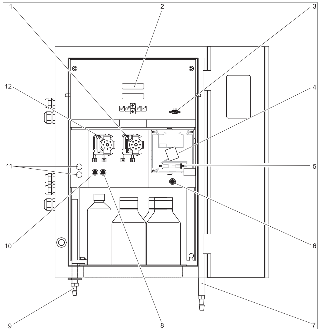
Fig. 1: Analyser (Schrankschrankausführung, ohne Schläuche)
