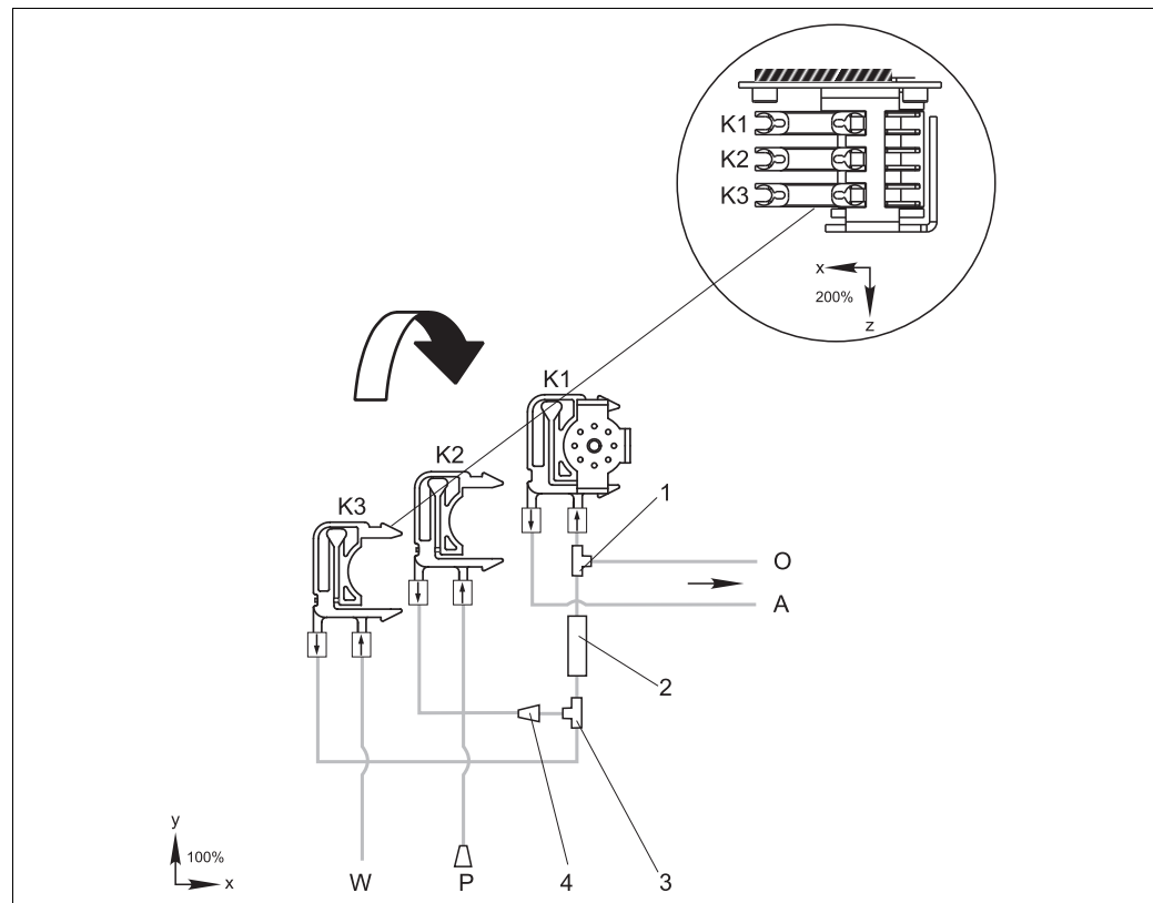
Fig. 21: Dilution module
