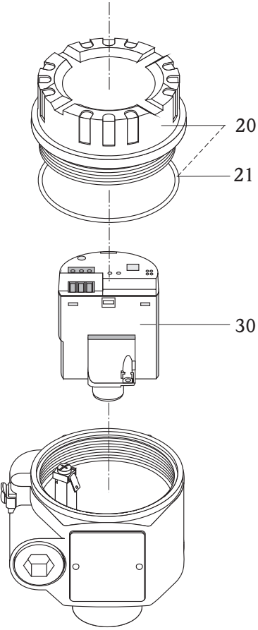
Aluminum housing (EEx d) F13 Aluminiumgehäuse (EEx d) F13
