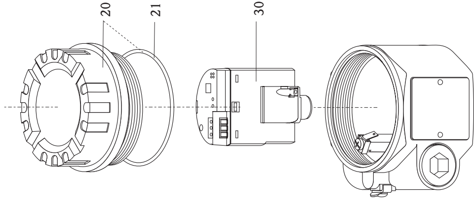
Aluminum housing F17 Aluminiumgehäuse F17
