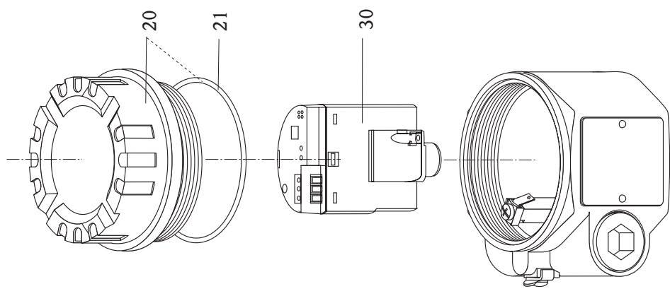
Aluminum housing F17 Aluminiumgehäuse F17
