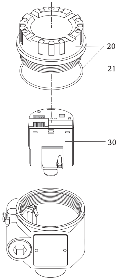
Aluminum housing (EEx d) F13 Aluminiumgehäuse (EEx d) F13
