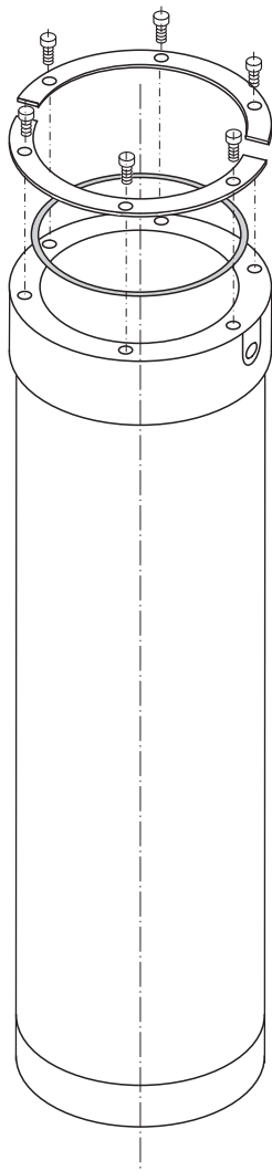
Accessory: cooling tube Zubehör: Wasserkühlmantel
