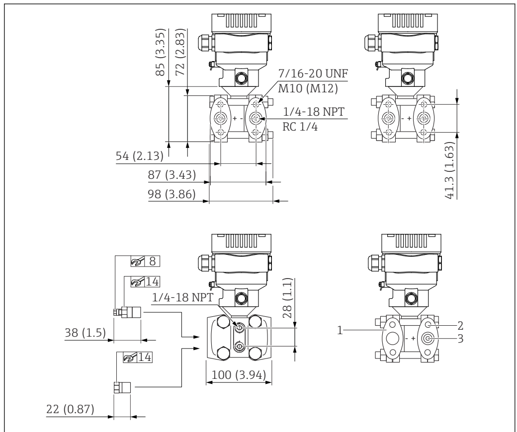
6 Vue de face, vue du côté gauche, vue du côté droit. Les écrous se trouvent toujours du côté négatif. Unité de mesure mm (in)
