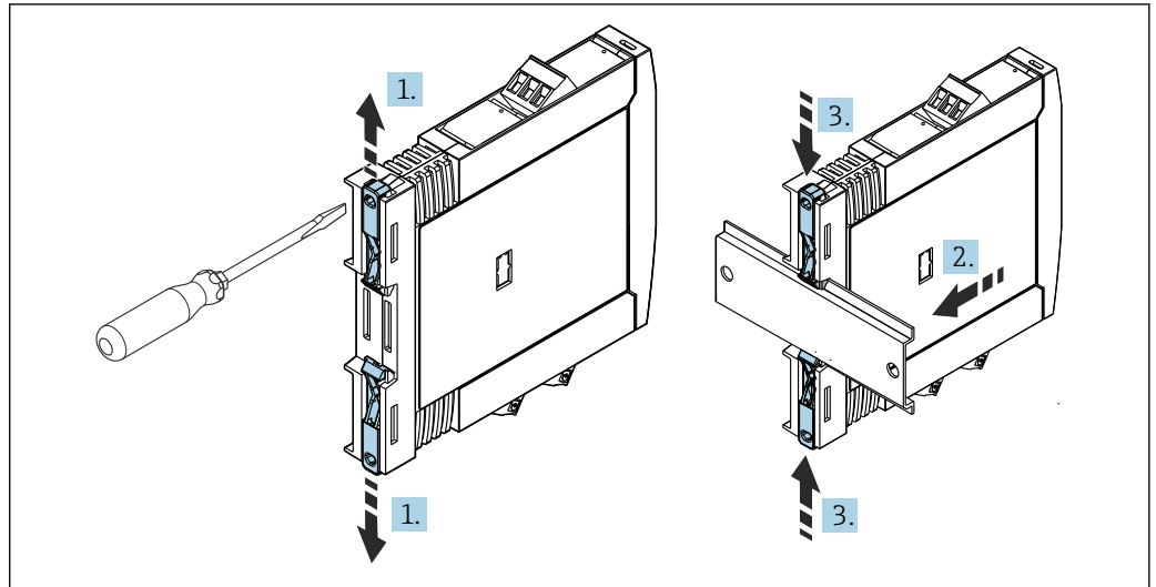
图 10 安装 DIN 导轨盘装型变送器
