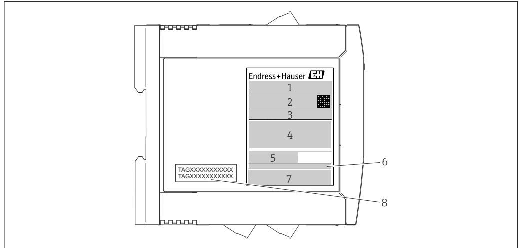
图 2 DIN 导轨盘装型温度变送器的铭牌示例（图例为防爆型仪表的铭牌）
