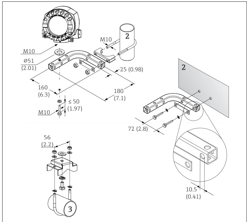
图 6 使用特殊安装支架安装现场型外壳，参见章节“附件”。外形尺寸 (mm (in))
