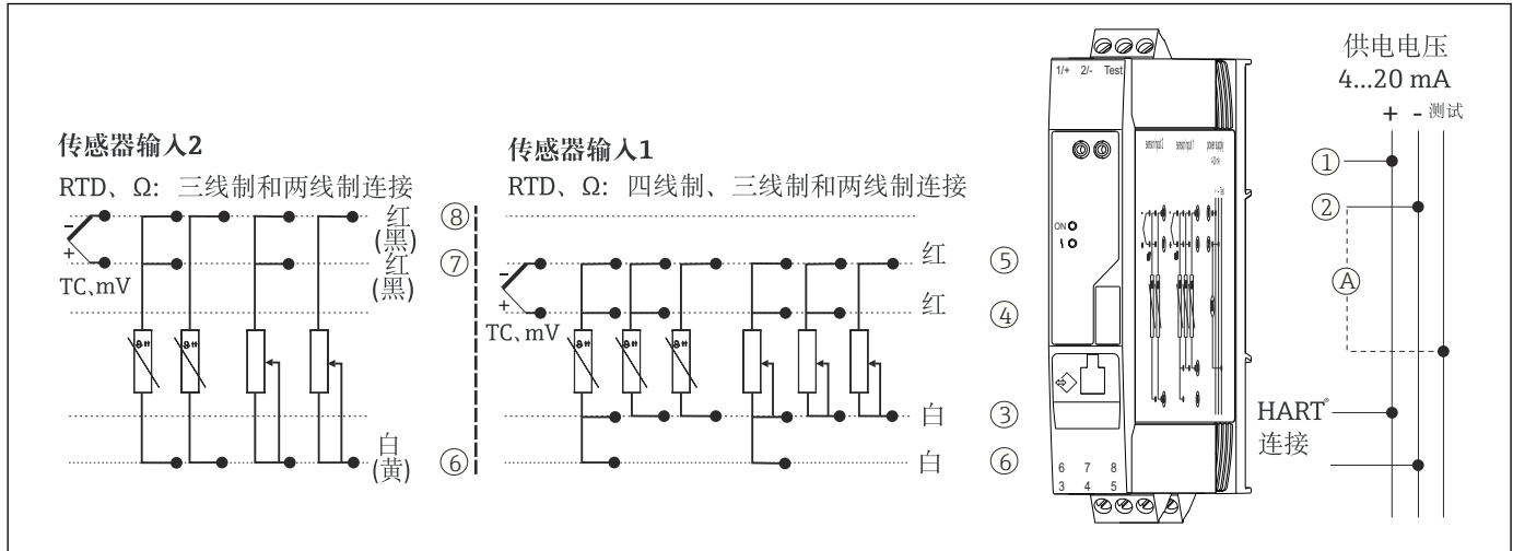
图 13 DIN 导轨盘装型变送器的接线端子分配
