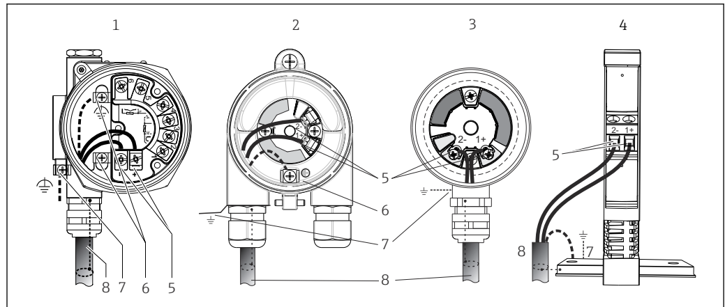
图 15 连接信号电缆和供电电缆
