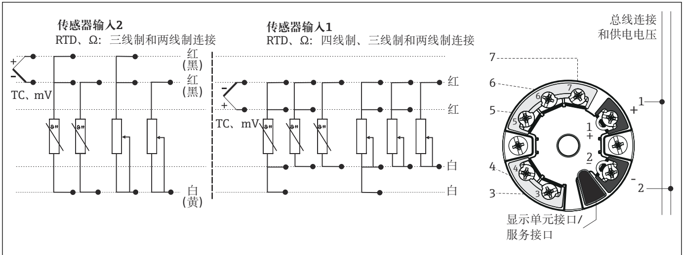
图 11 模块化变送器的接线端子分配
