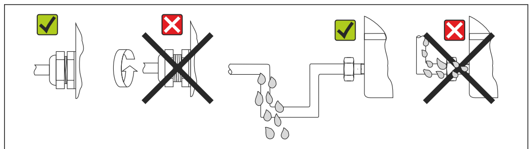
图 17 符合 IP67 防护等级的接线说明
