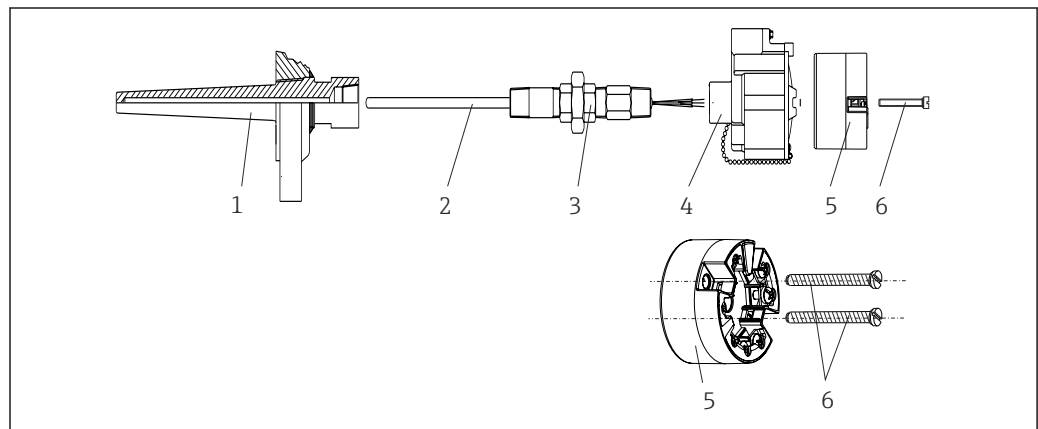
图 7 安装模块化变送器
