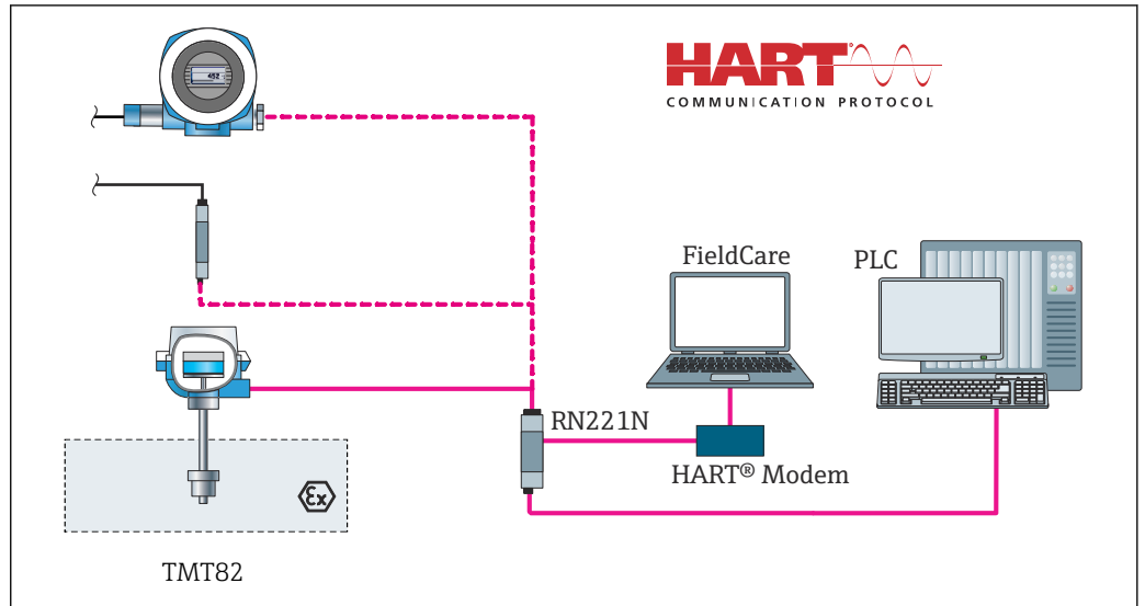
图 18 通过 HART®通信操作变送器
