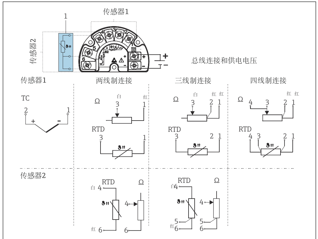
图 12 带有独立接线腔的现场型外壳的接线端子分配示意图
