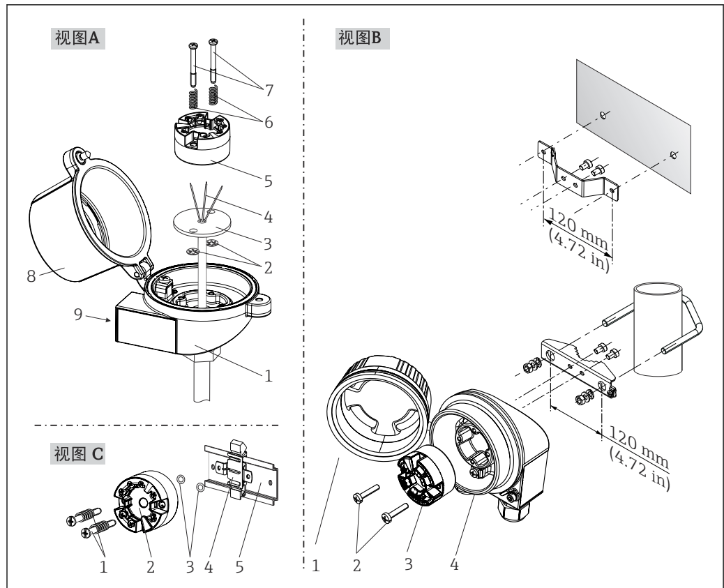
图 4 模块化变送器的安装示意图（三种安装方式）
