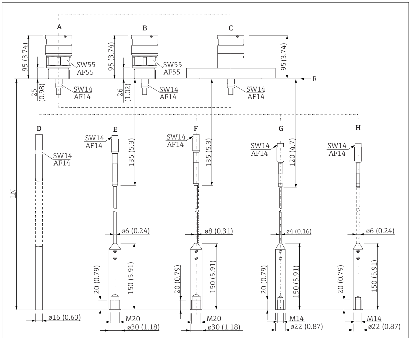
34 FMP57 : Raccord process / sonde. Unité de mesure mm (in)
