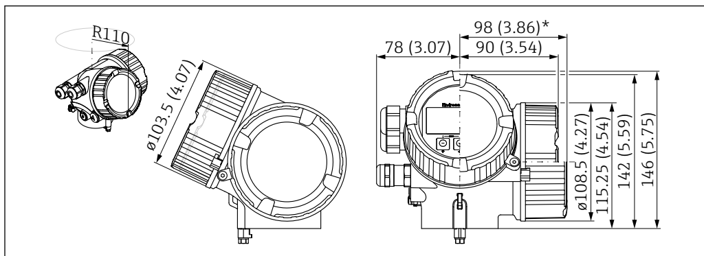
28 Boîtier GT18 (316L) ; dimensions en mm (in)
