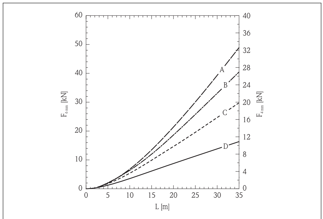
24 Ciment dans un silo métallique avec parois lisses ; charge de traction en fonction du niveau L pour des diamètres de câble de 6 mm (0,24 in) et 4 mm (0,16 in)
