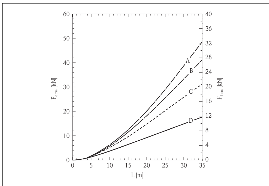
21 Sable dans un silo métallique avec parois lisses ; charge de traction en fonction du niveau L pour des diamètres de câble de 6 mm (0,24 in) et 4 mm (0,16 in)
