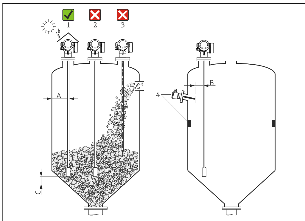
20 Conditions de montage pour Levelflex
