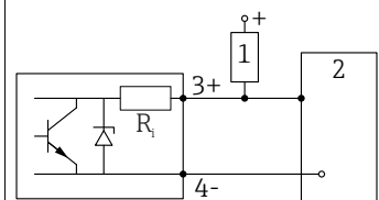
16 Raccordement à une entrée numérique
