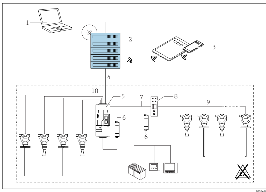
42 Exemple de plateforme de gestion des stocks avec SupplyCare Enterprise SCE30B
