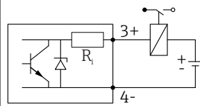
15 Raccordement d'un relais
