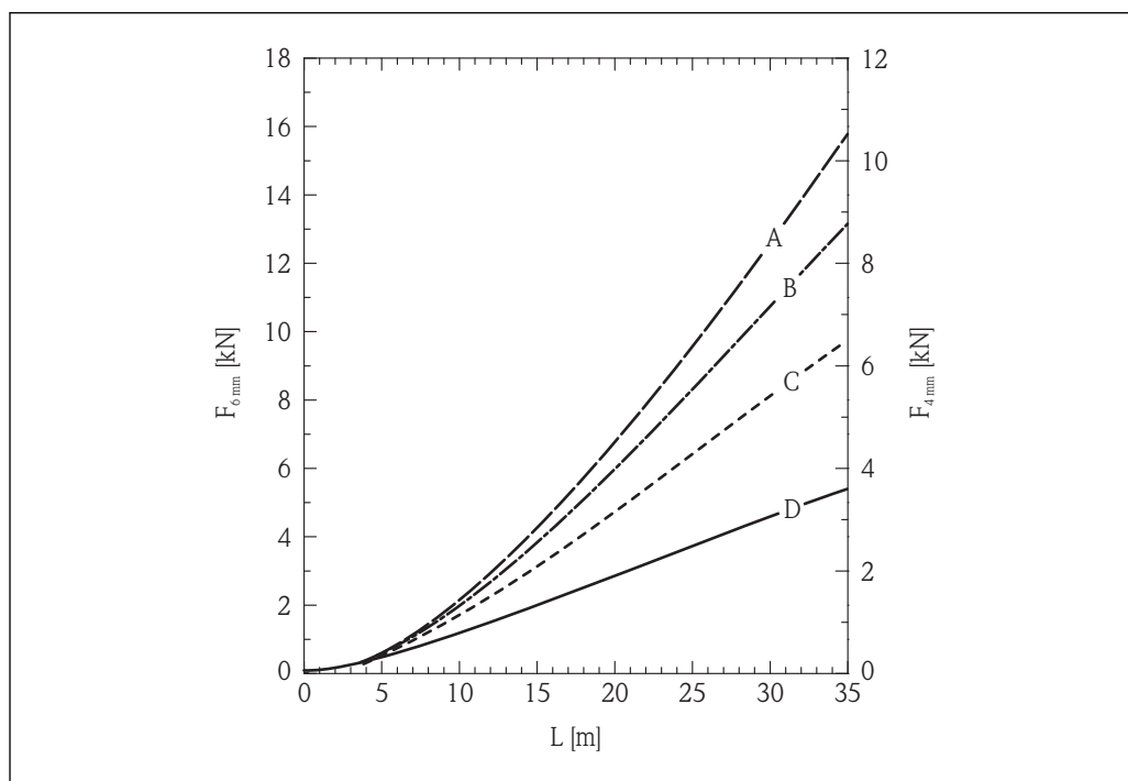
22 Granulés de polyéthylène dans un silo métallique avec parois lisses ; charge de traction en fonction du niveau L pour des diamètres de câble de 6 mm (0,24 in) et 4 mm (0,16 in)
