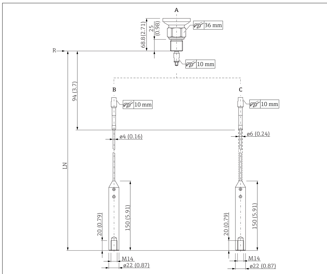
33 FMP56 : Raccord process / sonde. Unité de mesure mm (in)
