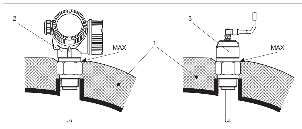
26 Raccord process avec filetage - FMP56, FMP57
