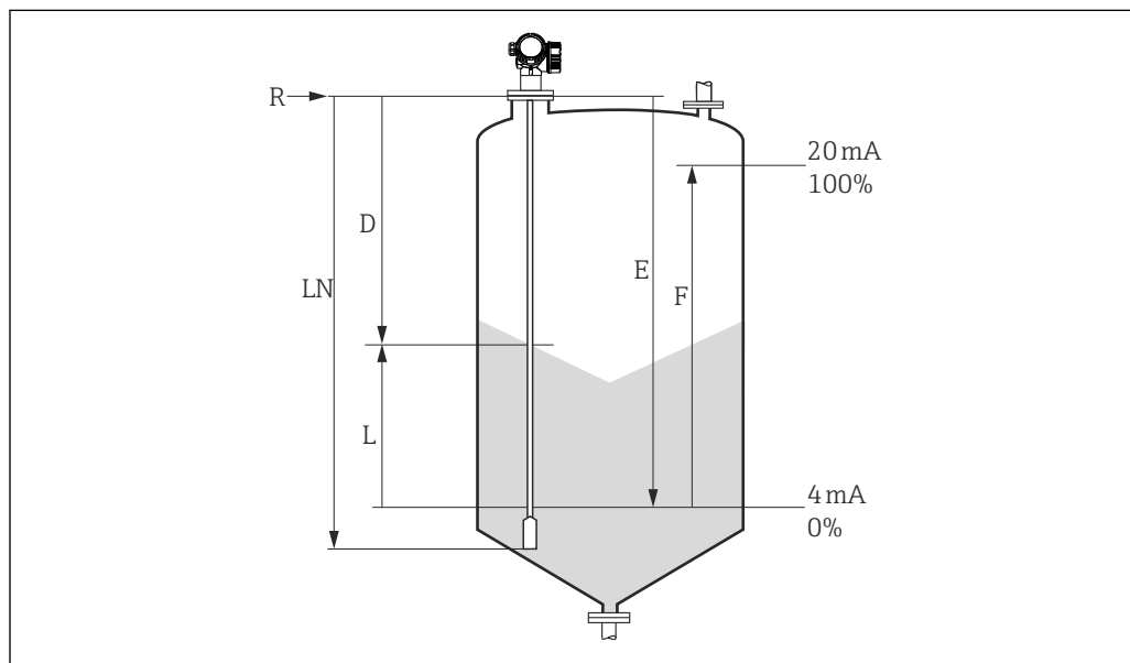
1 Paramètres pour la mesure de niveau avec un radar filoguidé
