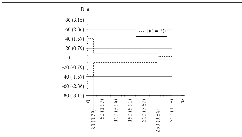
18 Ecart de mesure à l'extrémité de la sonde pour les sondes à câble
