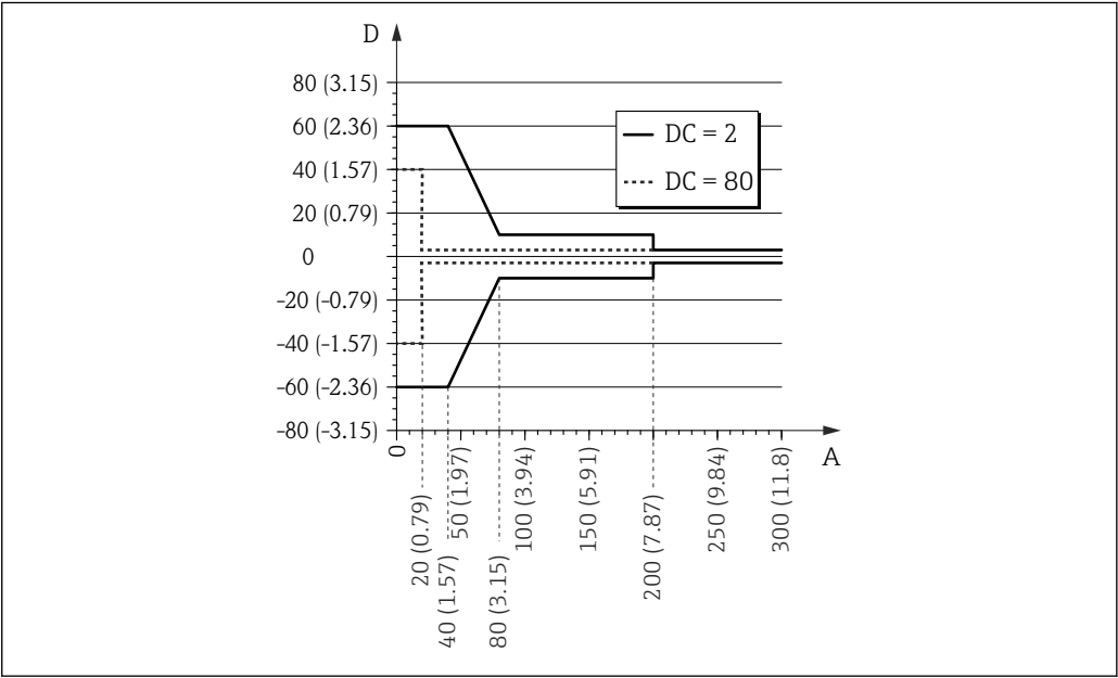
17 Ecart de mesure à l'extrémité de la sonde pour les sondes à tige et coaxiales A Distance de l'extrémité de la sonde [mm(in)] D Ecart de mesure : somme de la non-linéarité, la non-répétabilité et l'hystérésis
