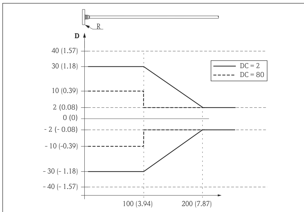
19 Ecart de mesure à l'extrémité supérieure de la sonde ; dimensions : mm (in)
