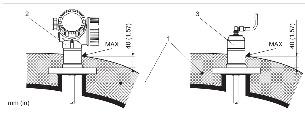
27 Raccord process avec bride - FMP57
